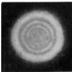
Fig. 1. Anelli di diffrazione prodotti su uno schermo opaco facendo passare la luce attraverso una cruna d'ago (N. R. Fowler).
