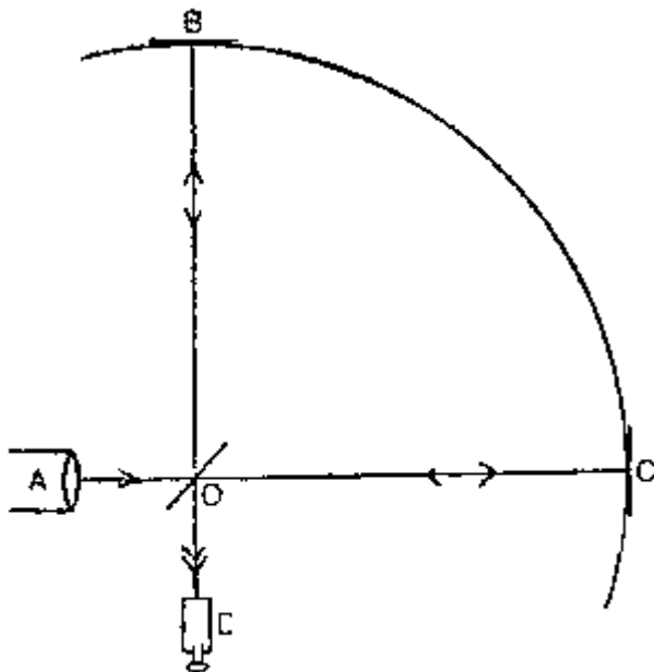
Fig. 1. - Diagramma per illustrare l'esperimento Michelson-Morley.
