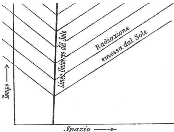
Fig. 3. - Diagramma per illustrare il moto del Sole e la sua radiazione nello spazio e nel tempo (cf. fig. 2).
