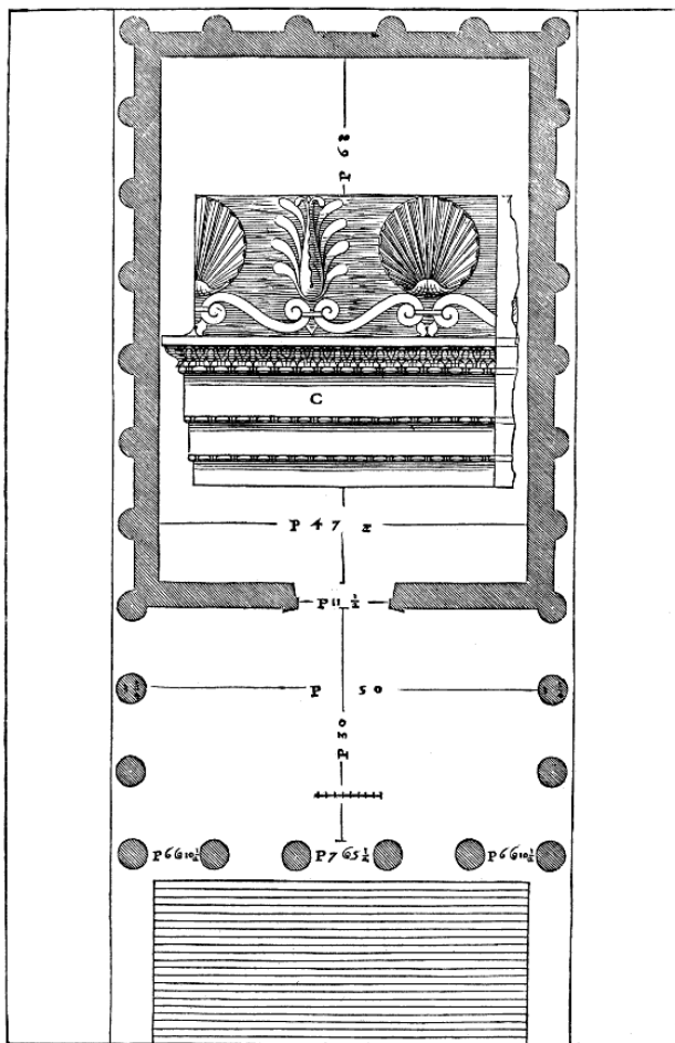
Tavola 92: 4-125.png Capitolo 30 – "Di questo tempio io ho fatto tre tauole. Nella Prima è disegnata la Pianta."
