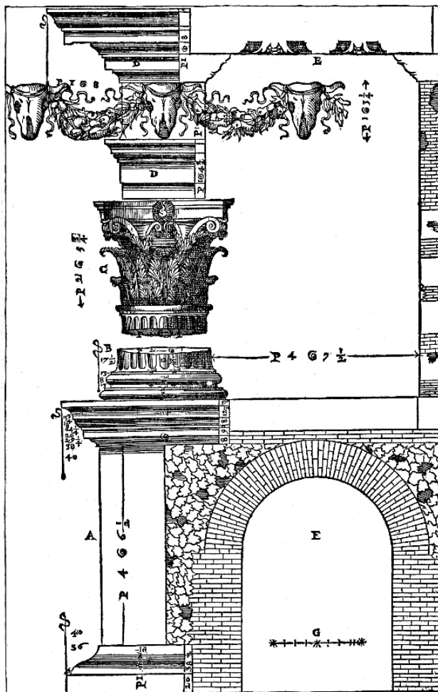
Tavola 66: 4-092.png Capitolo 23 – "Ho fatto di questo tempio quattro tauole. Nella Se- conda u'è l'Alzato."
