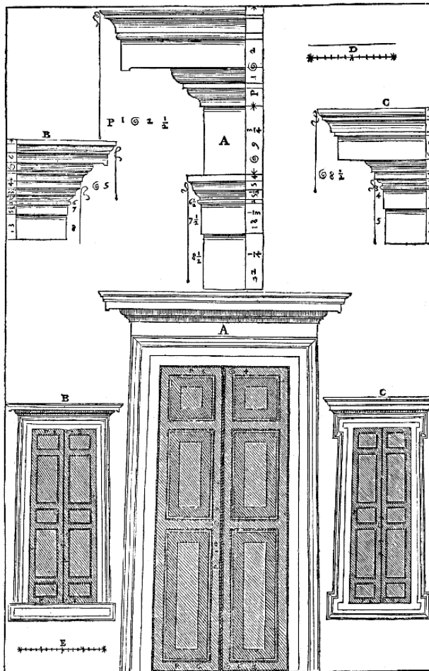
Tavola 67: 4-093.png Capitolo 23 – "Ho fatto di questo tempio quattro tauole. Nella Terza sono i membri del portico."
