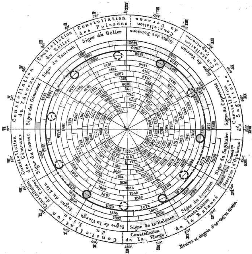
Fig. 238. – Moto di Giove in rapporto alla Terra.
