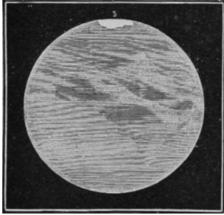
Fig. 58 – Velo atmosferico sul contorno interno del pianeta.
