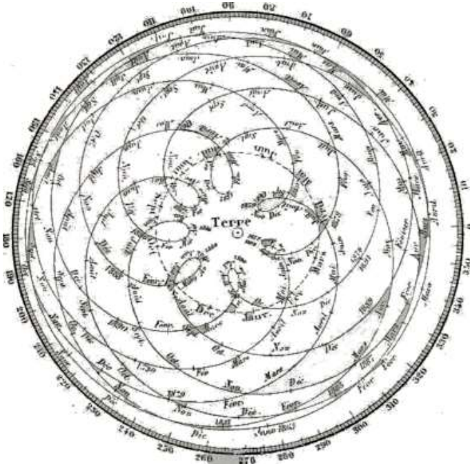
Fig. 103. – Movimento apparente di Venere in rapporto alla Terra.
