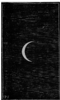
Fig. 112. – La Luna vista ad occhio nudo. Venere osservata col cannocchiale (4 febbraio 1883).
