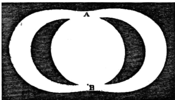
Fig. 291. – Disegno di Saturno fatto da BALL, nel 1665.
