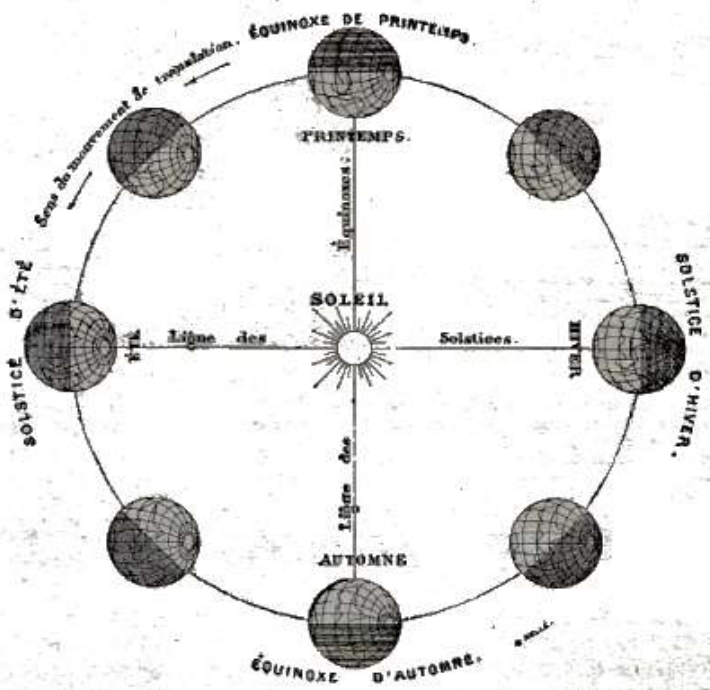
Fig. 119. – Movimento di Venere attorno al Sole e inclinazione dell'asse di rotazione.
