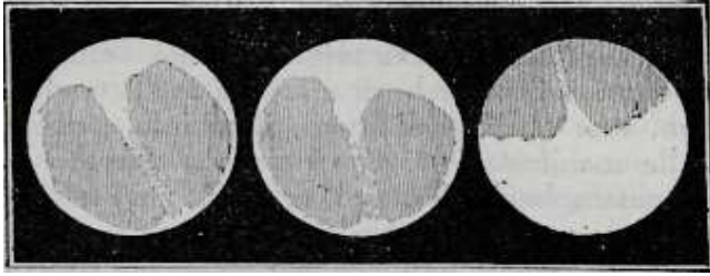
Fig. 266. – Aspetti osservati sul terzo satellite di Giove.
