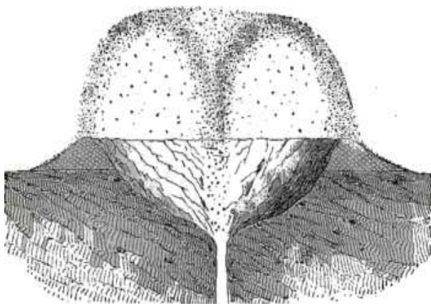
Fig. 213. – Sezione geologica d'un vulcano lunare nel suo periodo di massima attività.
