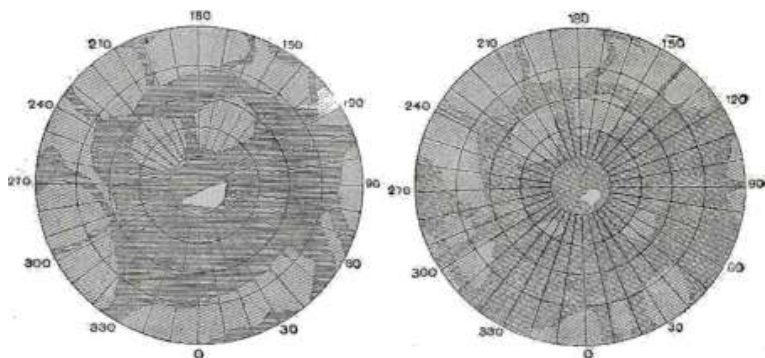
Fig. 53. – Nevi polari di Marte dopo le estati 1877 e 1879.
