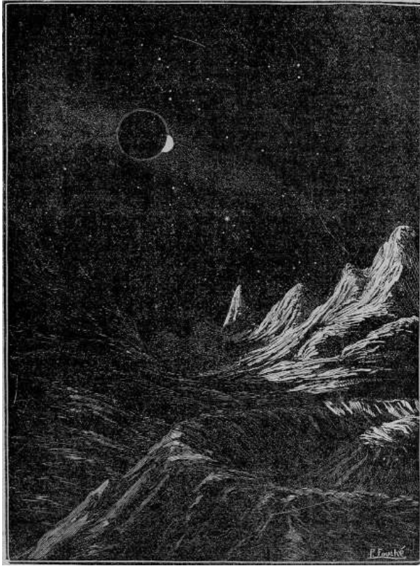
Fig. 230. – Nella Luna: Una eclissi di Sole causata dalla Terra.
