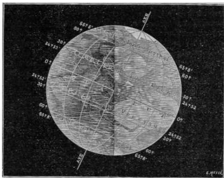
Fig. 49. – Inclinazione di Marte sul suo asse: le tre zone.
