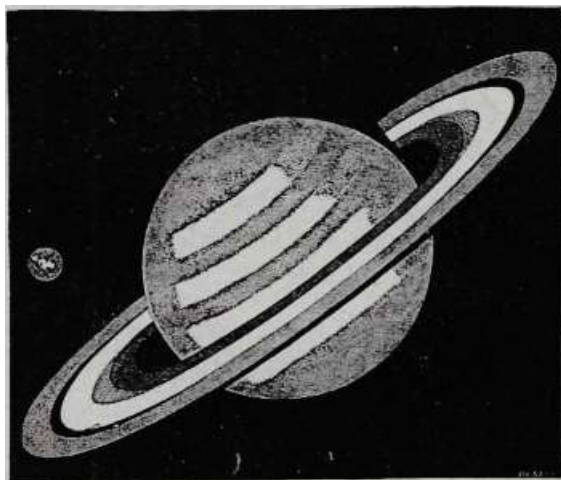
Fig. 282. – Grandezza comparata di Saturno e della Terra.
