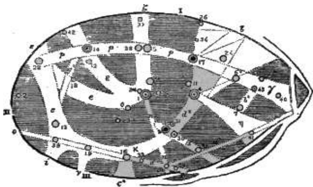
Fig. 223. – Planimetria del circo lunare Platone.
