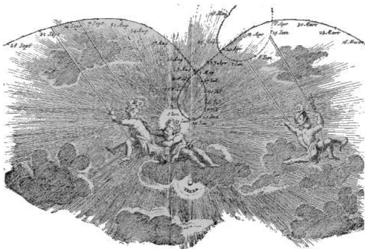
Fig. 157. – Le elongazioni di Venere e Mercurio da una parte e dall'altra del Sole. (Figura del XVIII secolo.)
