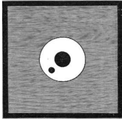
Fig. 78. – Una eclisse di Sole dovuto alle due Lune di Marte.
