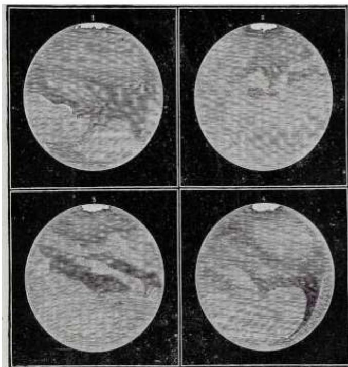
Fig. 16. – Aspetto di Marte nei giorni 1°, 29, 18 e 15 settembre 1877, rappresentante l'insieme del pianeta. dalla Machina Caelestis d'Hévélius (1673) 7 .
