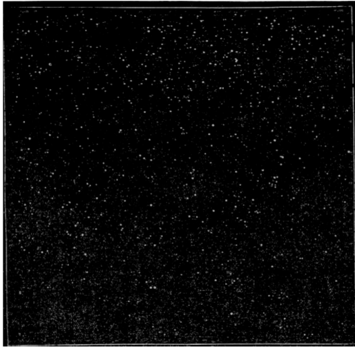
Fig. 234. – Carta delle stelle lungo l'eclittica.
