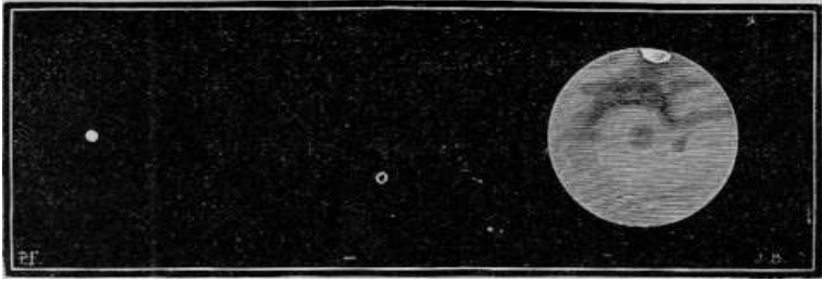
Fig. 74. — Prima osservazione fatta in Francia d'un satellite di Marte (27 agosto 1877).
