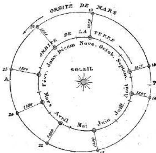
Fig. 39. – Ciclo delle opposizioni di Marte.
