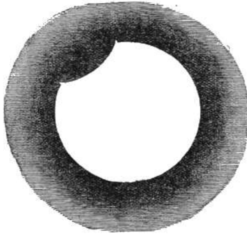
Fig. 218. – Punti osservati ai bordi della Luna durante una eclisse, il 29 settembre 1875.
