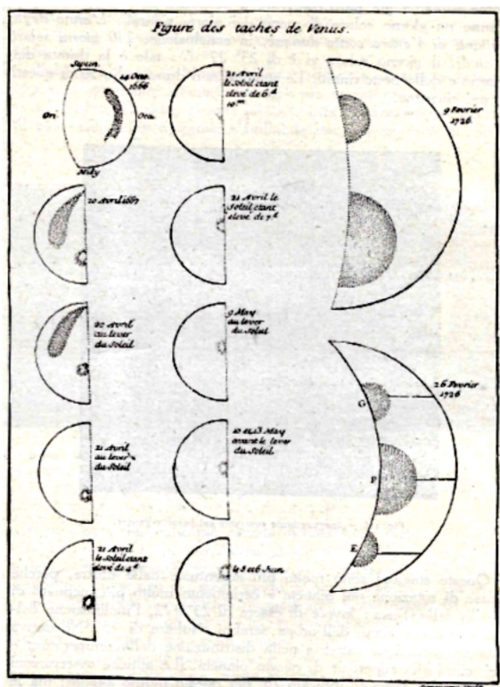
Fig. 115. – Osservazione delle macchie e della rotazione di Venere (Cassini, 1666-1667 e Bianchini, 1726).
