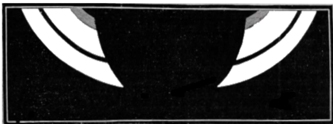
Fig. 307. – Gli anelli di Saturno e l'ombra del pianeta.
