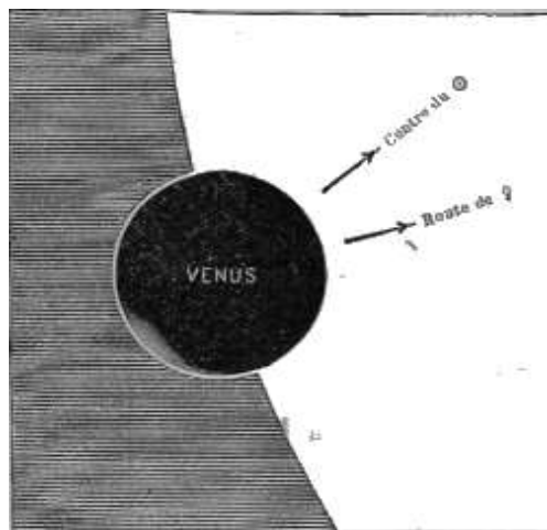
Fig. 138. – L'aureola atmosferica di Venere (Allegheny, 6 dicembre 1882)
