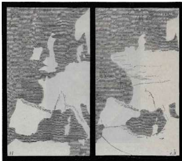
Fig. 27. – La Francia e le terre circostanti viste da lontano: 1. o con un cielo puro; 2. o con due strati di nuvole.
