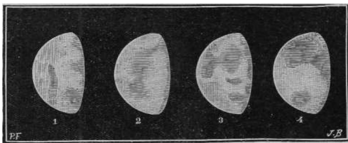
Fig. 125. – Aspetti geografici del pianeta Venere (De Vico, 1839).
