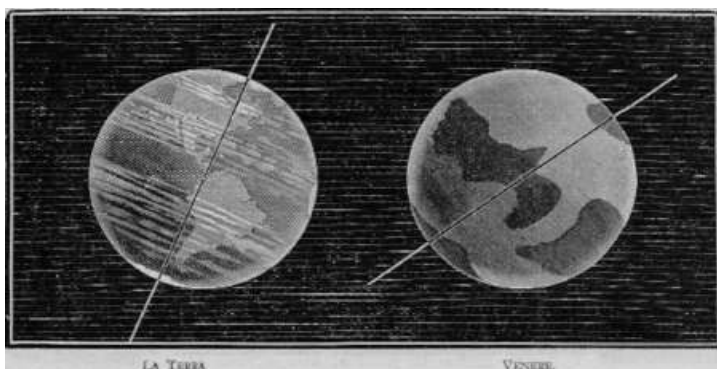
Fig. 117. – Inclinazione dell'asse di rotazione di Venere paragonata a quella della Terra.
