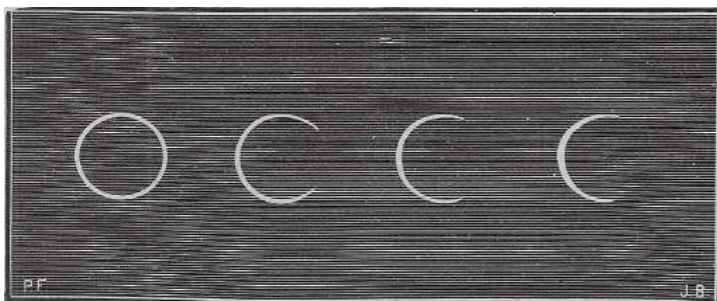
Fig. 140. – Venere vista sotto forma d'un anello luminoso.
