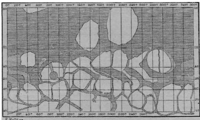
Fig. 67. – Carta di Marte fatta nel 1877 all’Osservatorio di Milano.
