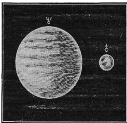
Fig. 321. – Grandezza comparata di Nettuno e della Terra.
