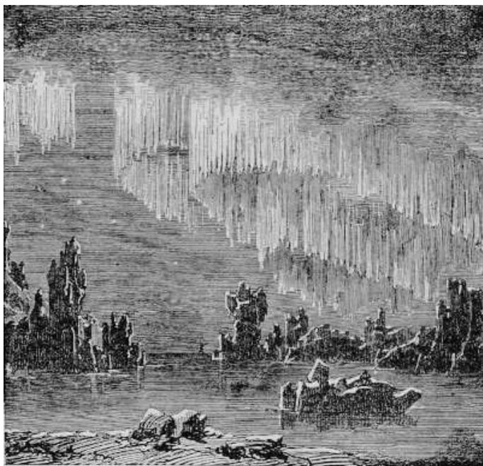
Fig. 190. – Una aurora boreale.
