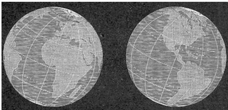
Fig. 22. – La Terra vista dallo spazio (dalla parte del Sole: 20 aprile a mezzogiorno e alle sei di sera).
