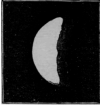
Fig. 164. – Fase di Mercurio. Troncatura del corno australe.
