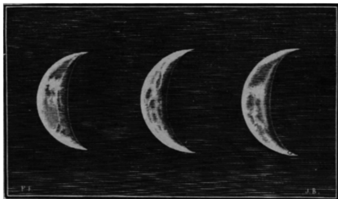
Fig. 127. – Aspetti geografici del pianeta Venere. (Disegni di Denning, 1881.)
