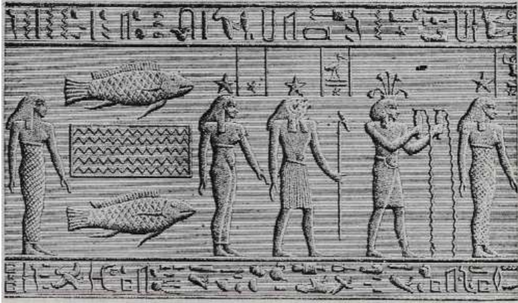
Fig. 273. – Zodiaco di Dendérah: Pianeti e costellazioni (seguito).
