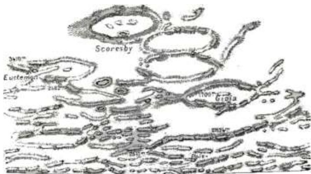
Fig. 208. – Il polo boreale della Luna, e le montagne dell'eterna luce (piano topografico).
