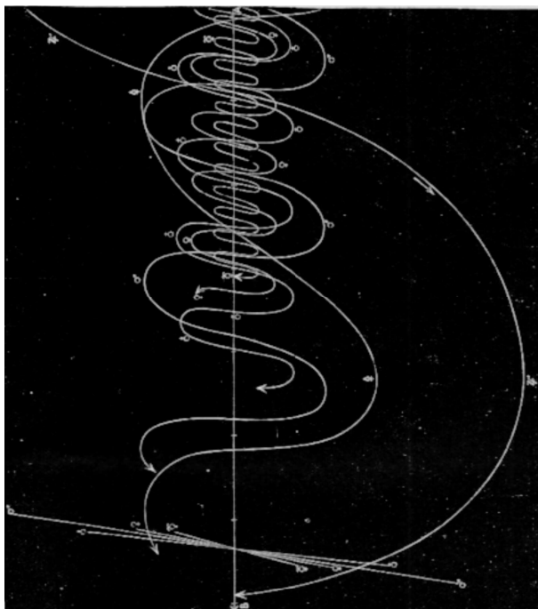
Fig. 185. – Eliche percorse da Giove, Vesta, Marte, la Terra, Venere e Mercurio nel loro moto annuale intorno al Sole.
