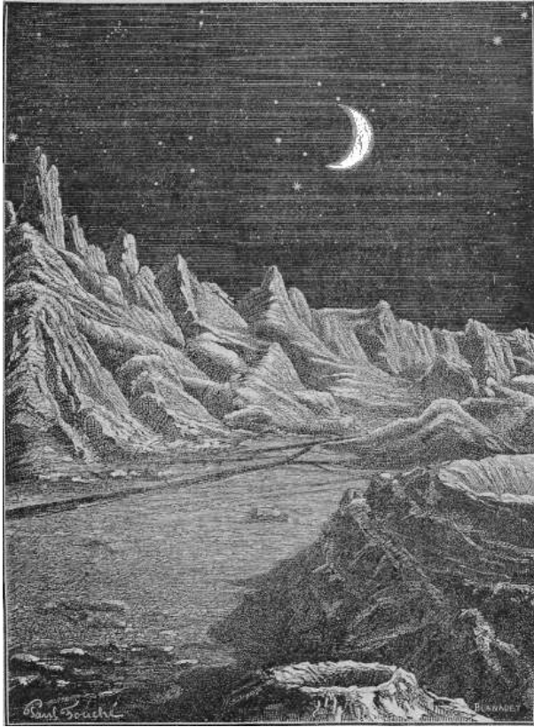
Fig. 229. – Fasi della Terra vista dalla Luna.
