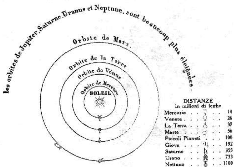
Fig. 8. – Pianta del sistema solare per i pianeti più vicini al Sole.
