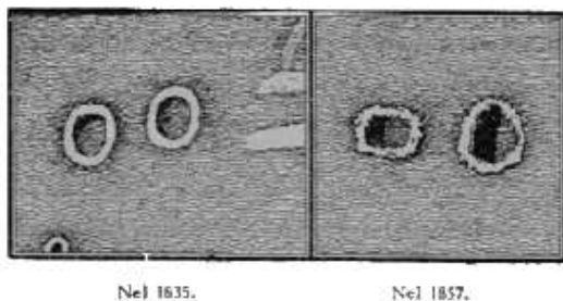
Fig. 221. – Il doppio cratere Messier.
