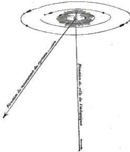
Fig. 184. – Caduta del sistema solare nello spazio.
