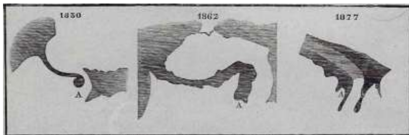
Fig. 24. – Variazioni osservate sul pianeta Marte: il golfo Kaiser e la Baia del Meridiano nel 1830, 1862 e 1877.
