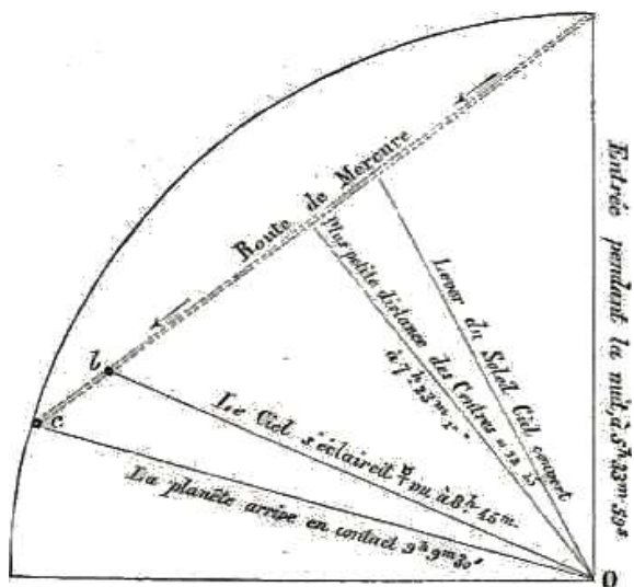
Fig. 154. – Quadrante nord-ouest del Sole, con indicazione del percorso seguito da Mercurio davanti al Sole.
