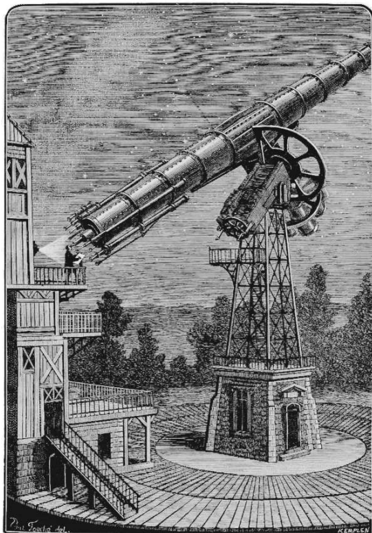
Fig. 2 – ... Esaminando con cura il pianeta ravvicinato, l'astronomo distingue e disegna i continenti, le coste, le isole della geografia di Marte...
