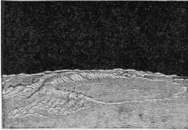
Fig. 215. – Circo sepolto alla riva dell’Oceano delle Tempeste.
