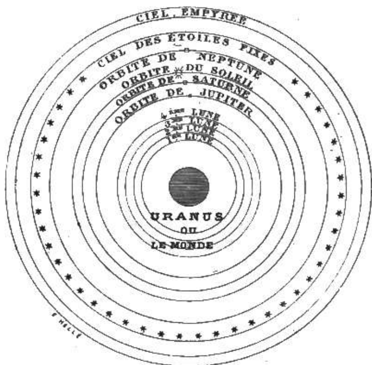
Fig. 318. – Il sistema del mondo per gli abitanti di Urano.
