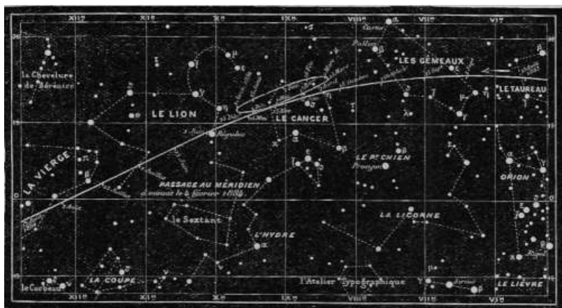
Fig. 41. – Cammino e posizioni del pianeta Marte sulla sfera celeste nell'anno 1883.
