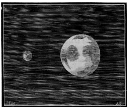
Fig. 118. – Osservazione problematica del satellite di Venere (Cassini, 1672).
