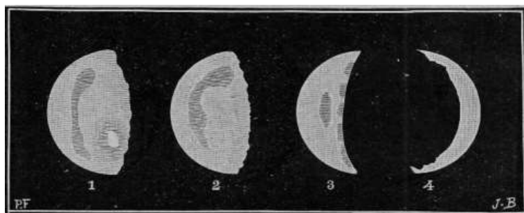
Fig. 126. – Aspetti geografici del pianeta Venere (1, Cassini, 1666; 2, 3 e 4, Langdon, 1871).
