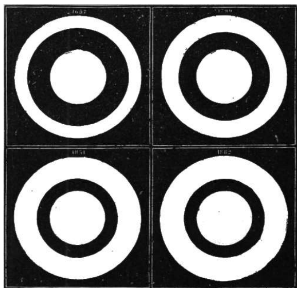
Fig. 297. – Diagrammi delle misure degli anelli di Saturno in 225 anni.
