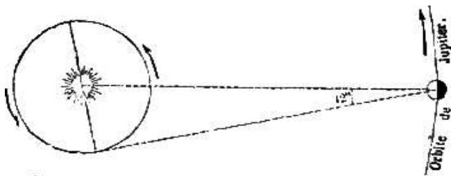
Fig. 257. – Relazione tra l'orbita di Giove e quella della Terra.
