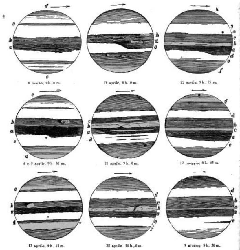
Fig. 249. – Aspetti telescopici di Giove, presi nel 1874.
