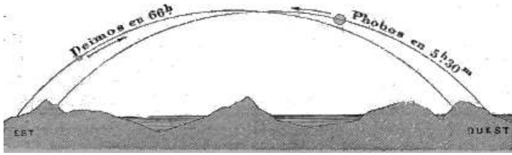
Fig. 75. – Cammino dei satelliti di Marte nel cielo del loro pianeta.
