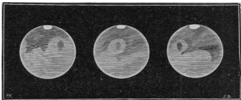
Fig. 48. – Come si osserva la rotazione diurna di Marte.
