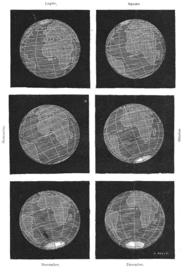
Fig. 183. – Posizioni della Terra dinanzi alla luce solare, a mezzogiorno, durante i dodici mesi dell'anno.
