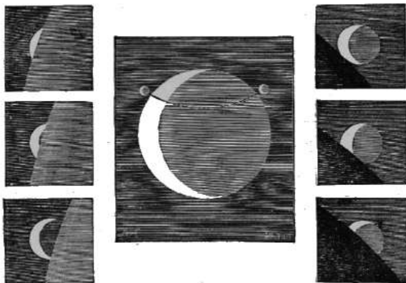
Fig. 107. – Occultazione di Venere dalla Luna (il 14 ottobre 1874).
