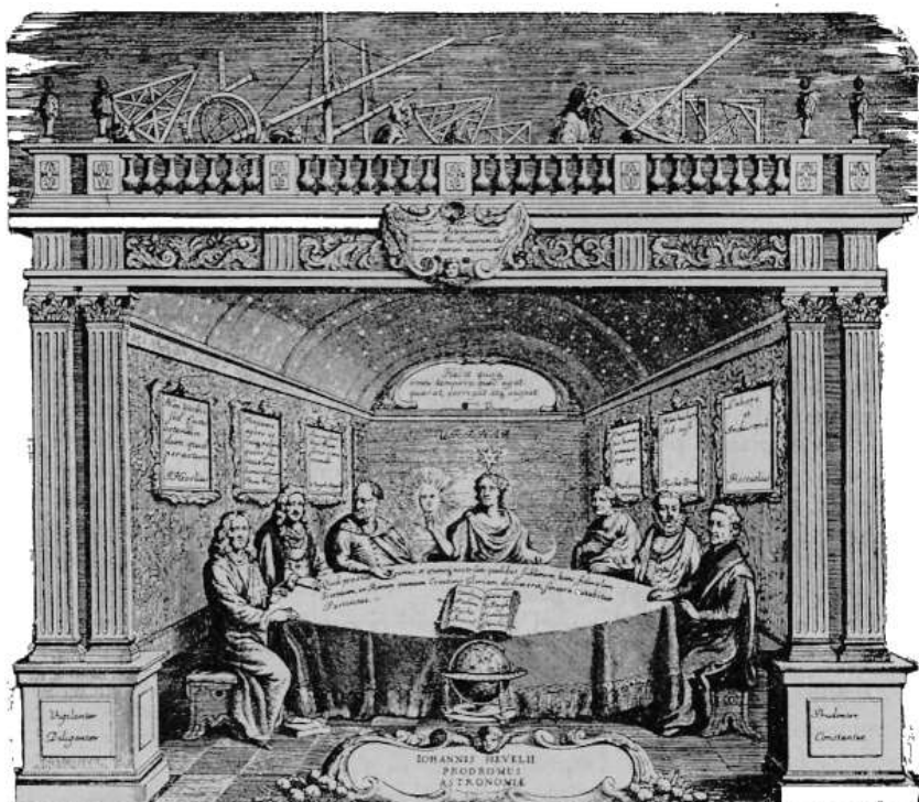
Fig. 301. – Cenacolo d'astronomi presieduto da Urania (Hévélius, 1690).
