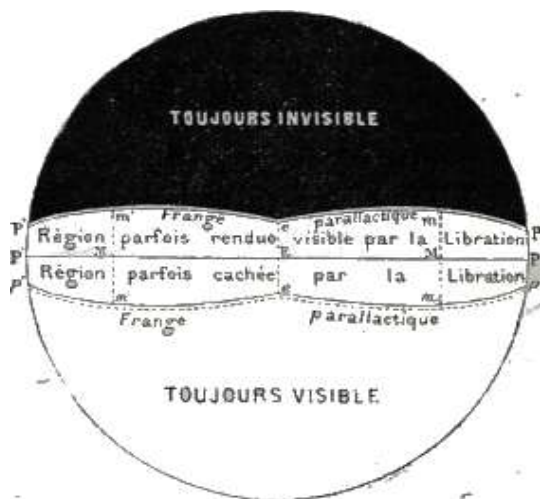
Fig. 198. – Superficie del globo lunare che noi conosciamo.
