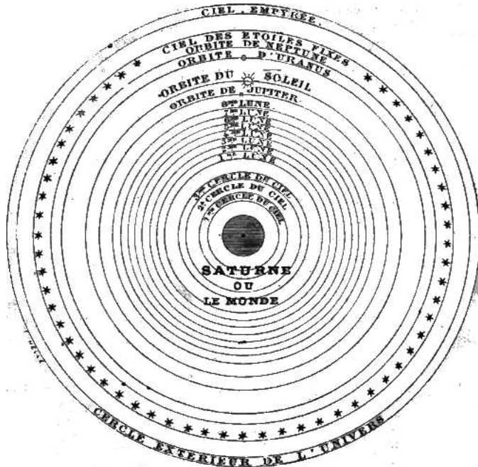
Fig. 310. – Il sistema del mondo visto da Saturno.
