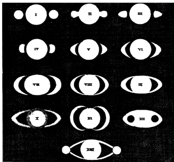
Fig. 285. – Prime rappresentazioni di Saturno.
