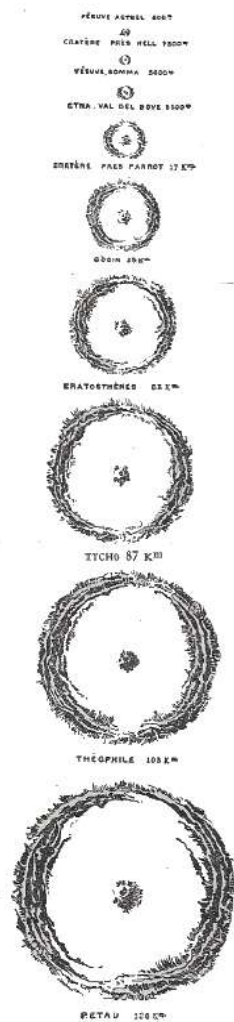
Fig. 210. – Dimensioni dei crateri lunari.
