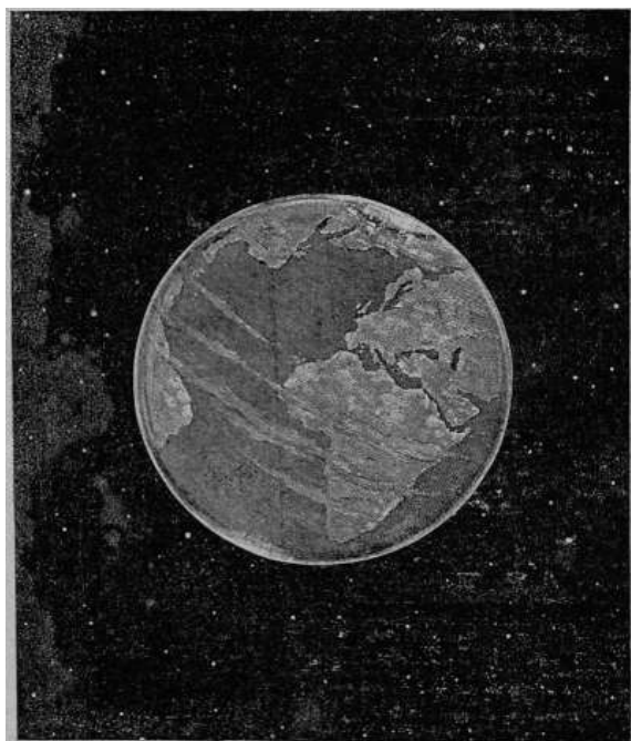
Fig. 231. – La Terra piena vista dalla Luna.
