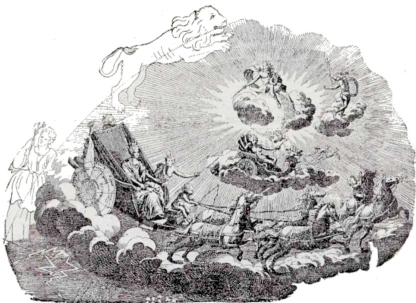
Fig. 104. – La Terra accompagnata dalla Luna, Venere e Mercurio, giganti intorno al Sole (Figura del XVIII secolo).
