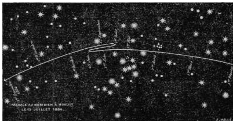
Fig. 146. – Cammino del pianeta Terra nel cielo degli abitanti di Venere.
