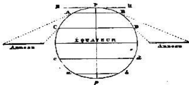
Fig. 303. — Sezione geometrica attraverso Saturno e i suoi anelli.
