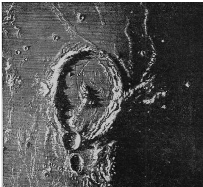
Fig. 207. – La montagna lunare Gassendi, al levar del sole.
