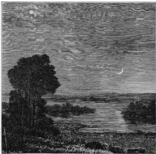
Fig. 77. – Le due Lune di Marte.
