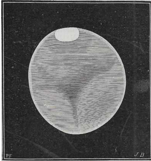
Fig. 10. – Aspetto telescopico del pianeta Marte, in un istrumento di media potenza.
