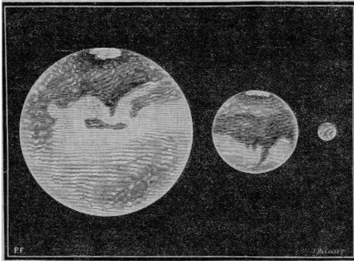
Fig. 44. – Dimensioni apparenti di Marte alle sue distanze estreme e medie. (Scala da 2 mm. a 1").
