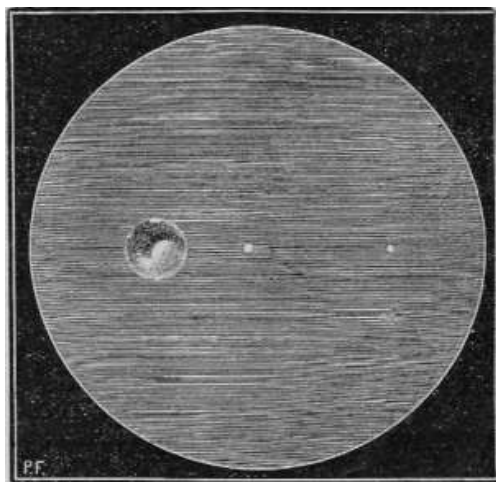
Fig. 72. – Marte e i suoi due satelliti.
