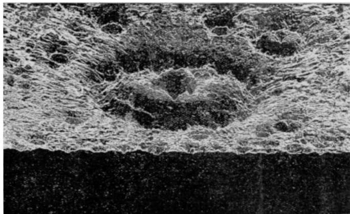
Fig. 209. – Tipo delle montagne lunari.
