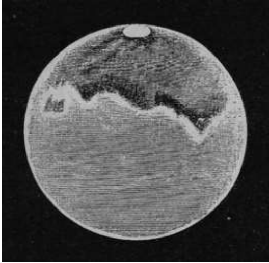
Fig. 64. – Meteorologia di Marte: tracce di nubi lungo le coste.
