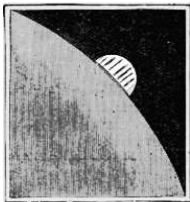
Fig. 217. – Giove occultato dalla Luna, il 24 maggio 1860.
