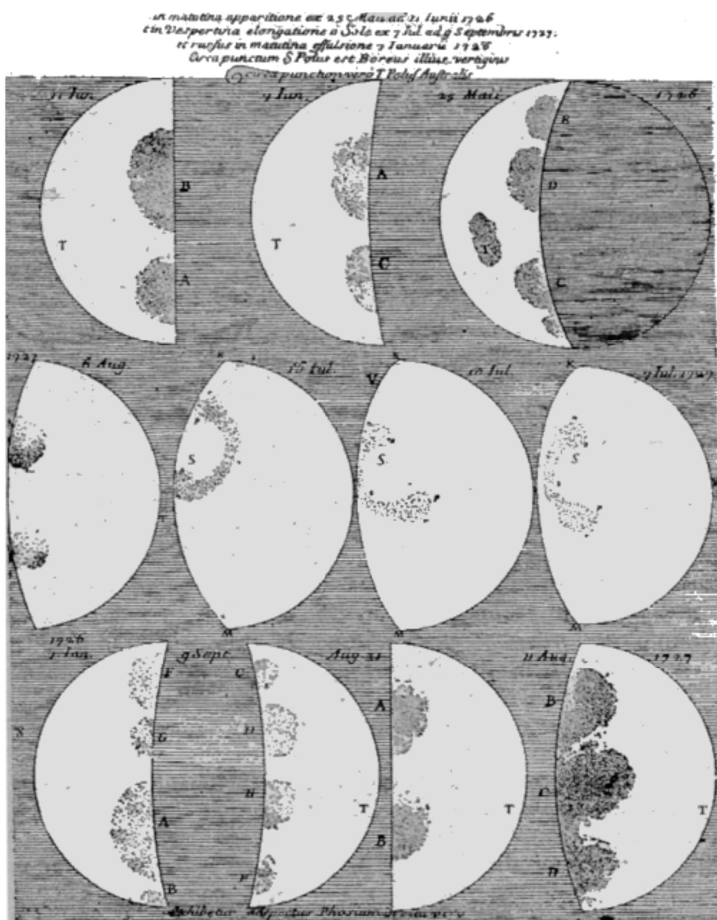
Fig. 122. – Disegni del pianeta Venere fatti nel 1726-27, da Bianchini, col mezzo di un cannocchiale di 30 metri.
