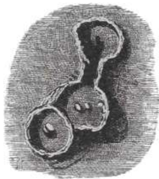
Fig. 205. – Le montagne lunari: Caterina, Cirillo e Teofilo.
