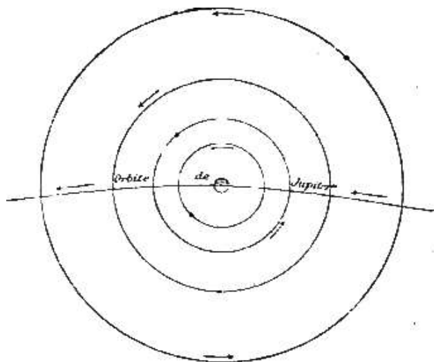
Fig. 265. – Il sistema di Giove: i suoi primi quattro satelliti.
