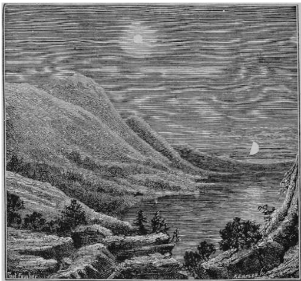
Fig. 260. – Le notti hanno sempre il chiaro di Luna e sono talvolta rischiarate da più Lune.
