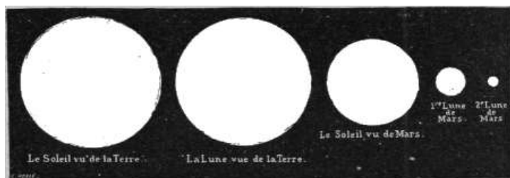
Fig. 76. – Grandezza apparente relativa del Sole e delle Lune di Marte.
