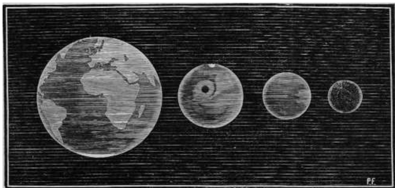
Fig. 45 – Grandezza comparata della Terra, Marte, Mercurio e la Luna.
