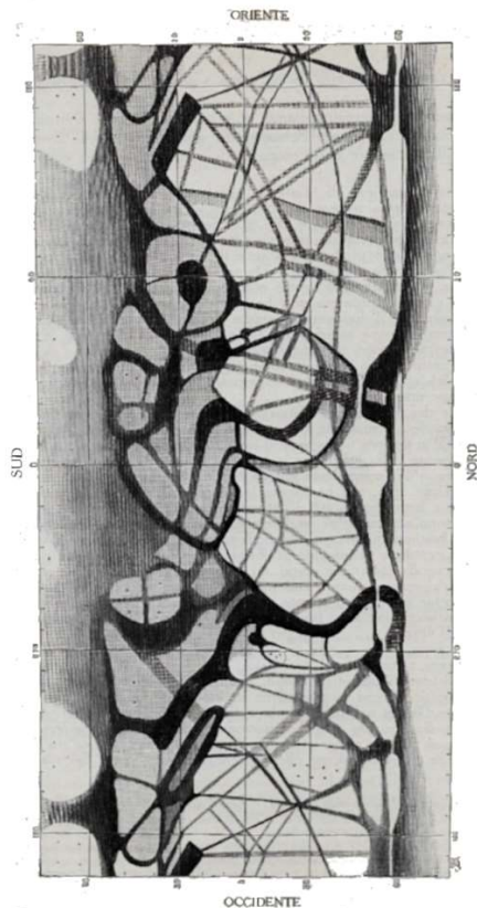
Fig. 30. – Canali enigmatici osservati nel pianeta Marte.
