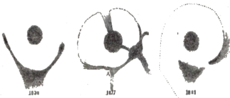
Fig. 26. – Variazioni osservate sul pianeta Marte. Il mare Daedalia nel 1830, 1877 e 1881.
