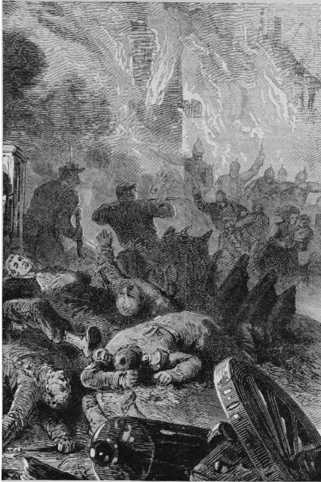
Fig. 192. – Il campo d'onore dell'umanità terrestre
