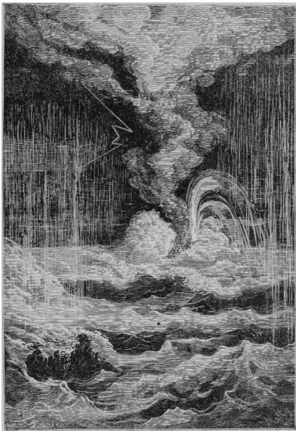
Fig. 256. – I vapori caldi s'innalzano e ricadono in pioggia... È la genesi di un mondo.
