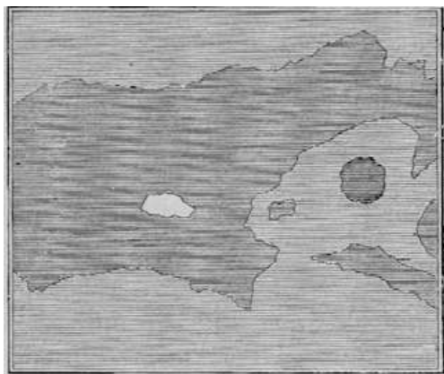
Fig. 62. – Frammento della geografia di Marte: L'isola nevosa .
