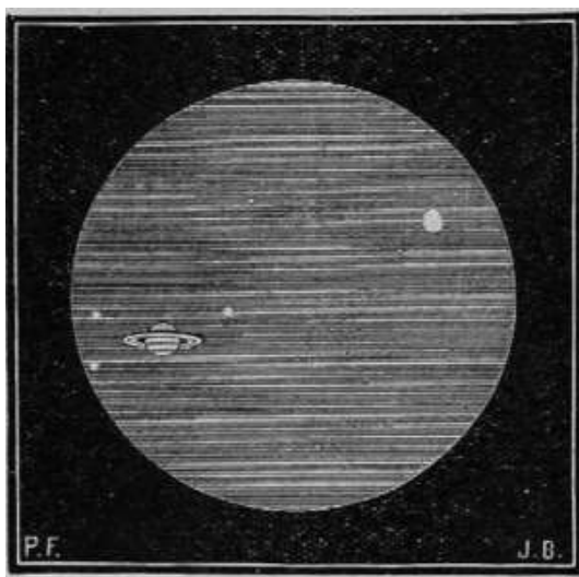
Fig. 42. – Congiunzione di Marte con Saturno il 1. o luglio 1879
