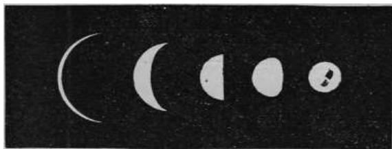
Fig. 163 – Le fasi di Mercurio.
