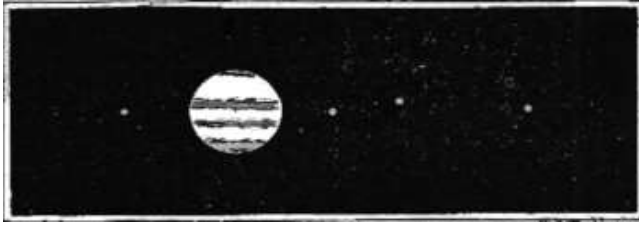
Fig. 262. – Giove ed i suoi primi quattro satelliti.
