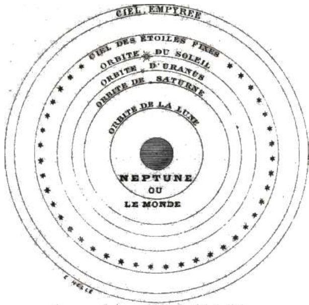
Fig. 324. – Il sistema del Mondo visto da Nettuno.
