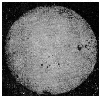
Fig. 105. — Aspetto delle macchie solari.
