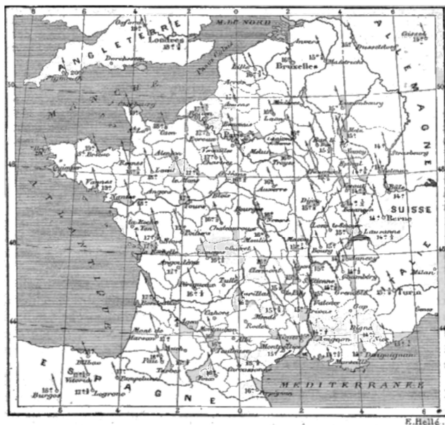
Fig. 189. – Declinazione dell'ago calamitato.
