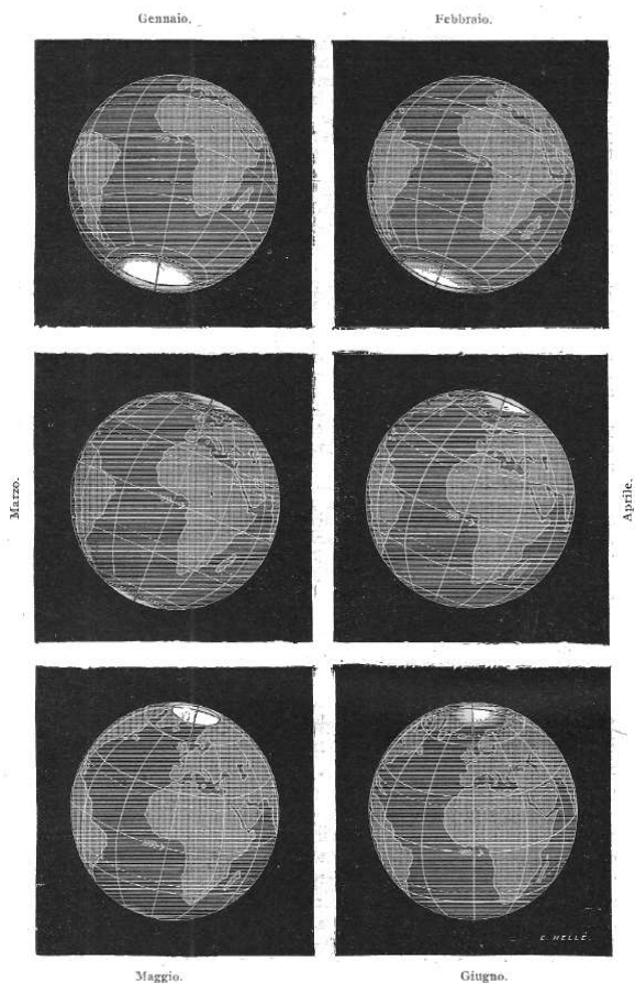
Fig. 182. – Posizioni della Terra dinanzi alla luce solare, a mezzogiorno, durante i dodici mesi dell'anno.
