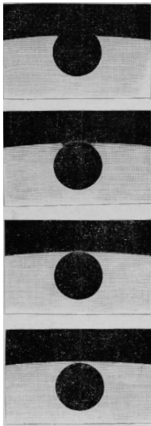
Fig. 139. – L'aureola atmosferica di Venere (Potsdam, 6 dicembre 1882).
