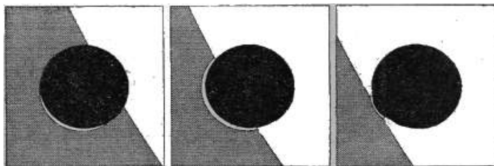
Fig. 136. – L'aureola atmosferica di Venere (Nizza, 6 dicembre 1882).
