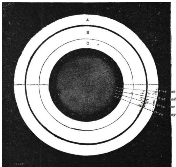
Fig. 295. – Il sistema di Saturno (misure di O. Struve, 1882).
