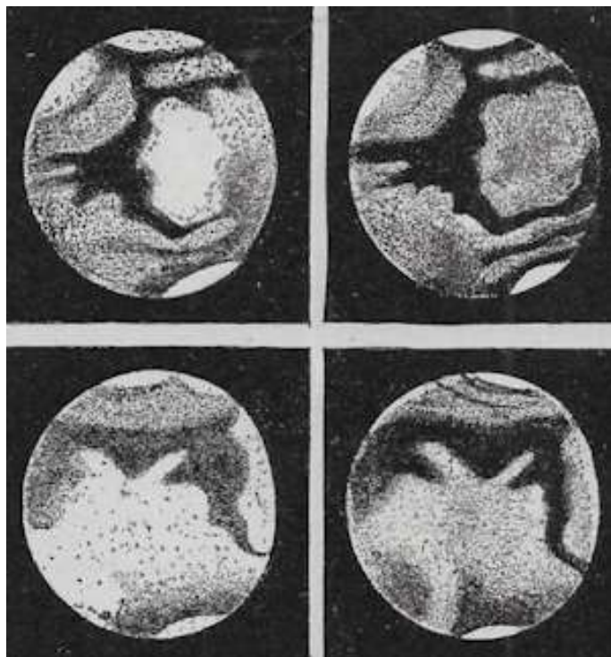
Fig. 13. – Aspetti di Marte il 13, 14, 17 e 18 giugno 1858.
