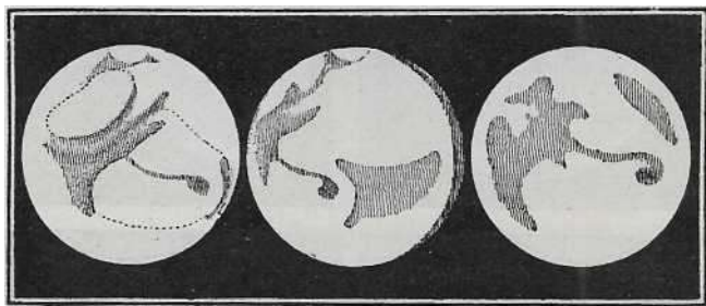
Fig. 11. – Aspetti di Marte, il 14 settembre e il 20 ottobre 1830, e il 16 dicembre 1832.
