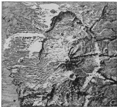
Fig. 212. – Il cratere terrestre di Teneriffa: Analogia notevole con i crateri lunari.
