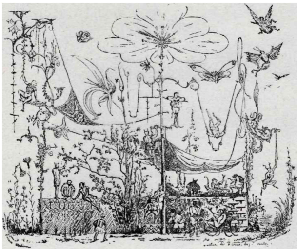
Fig. 84. – Scena immaginaria presso gli abitanti di Giove.
