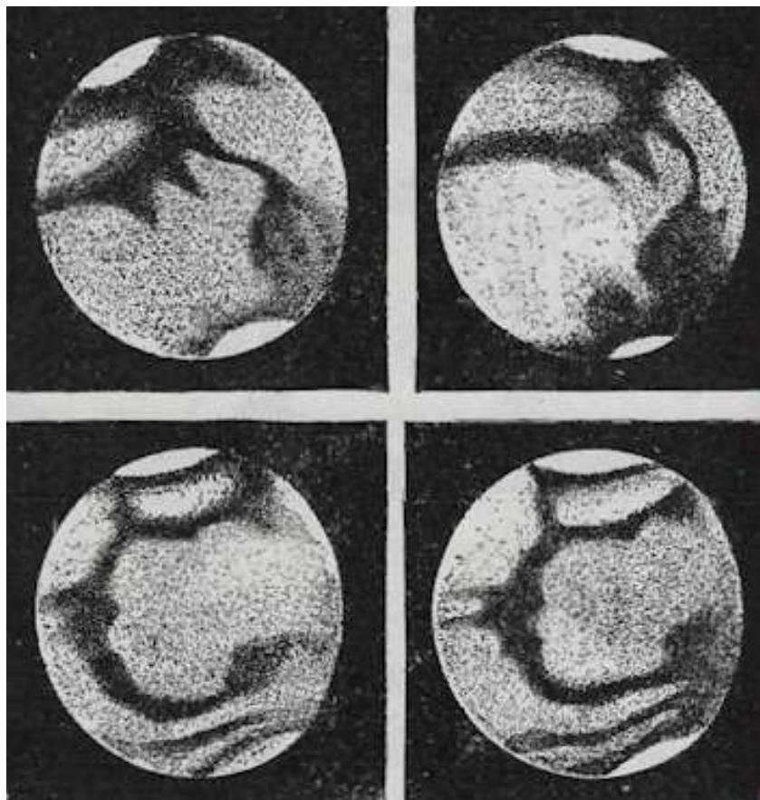
Fig. 12. – Aspetti di Marte il 5, 6, 7 e 10 giugno 1858.
