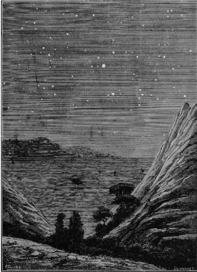
Fig. 149. – La Terra, vista da Venere, brilla nel cielo come una stella di prima grandezza.
