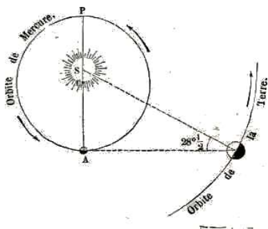
Fig. 152. — Relazione fra l'orbita di Mercurio e quella della Terra.
