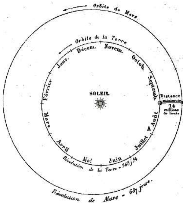
Fig. 9. – Rapporto fra l'orbita di Marte e quella della Terra.
