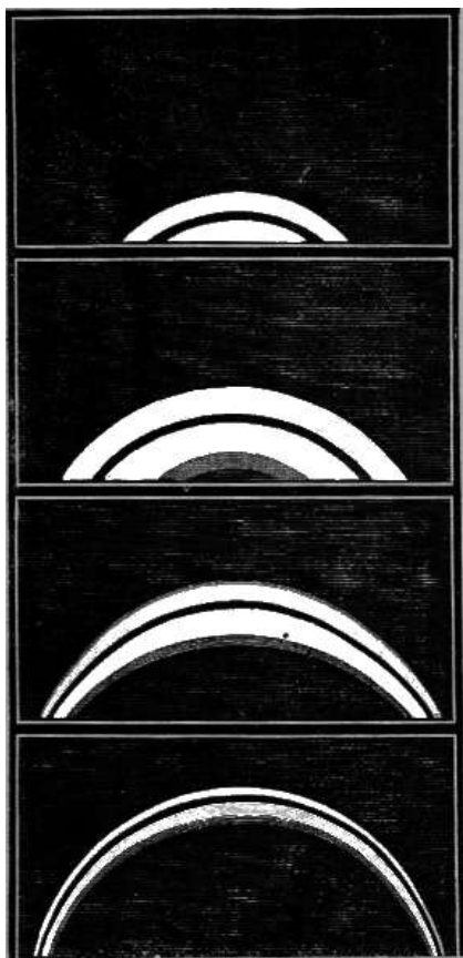
Fig. 304. – Aspetti degli anelli alle diverse latitudini del pianeta.
