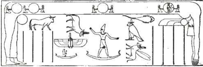
Fig. 277. – Bassorilievo astronomico nel soffitto del tempio di Ermotide.
