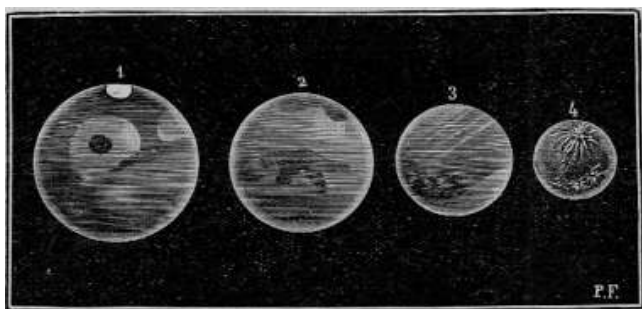
Fig. 172. – Grandezze comparate di Marte, Ganimede, Mercurio e la Luna
