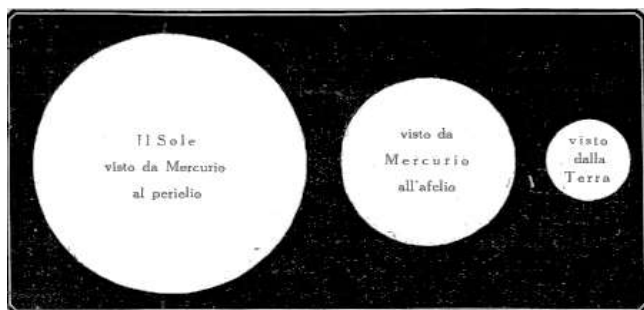
Fig. 170. – Grandezza comparata del Sole visto da Mercurio e dalla Terra.
