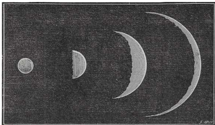
Fig. 109. – Grandezza comparata delle quattro fasi principali di Venere.
