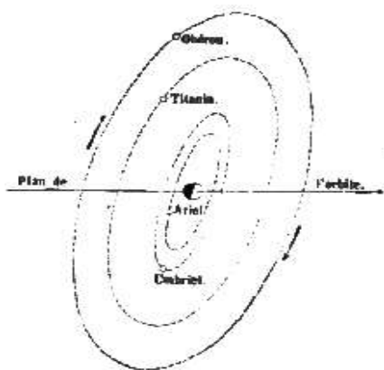
Fig. 316. — Il sistema di Urano.
