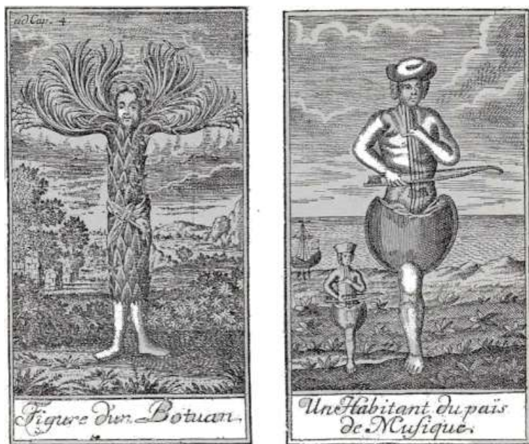
Fig. 174. – Esseri immaginari, da un viaggio nei pianeti (Holberg, 1741).
