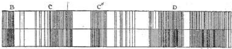
Fig. 59. — Righe atmosferiche dello spettro solare che si trovano nello spettro di Marte.
