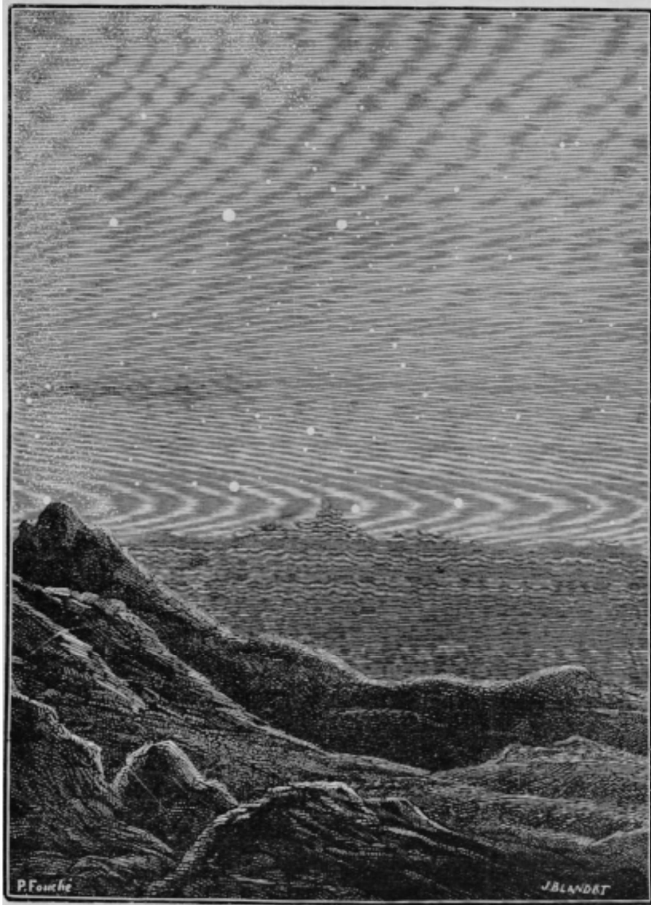
Fig. 177. – La Terra, stella dello Zodiaco, vista dal mondo di Mercurio.
