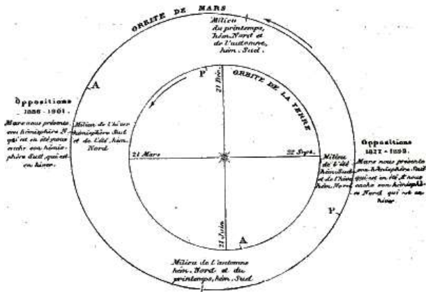
Fig. 52. – Le stagioni sul pianeta Marte.
