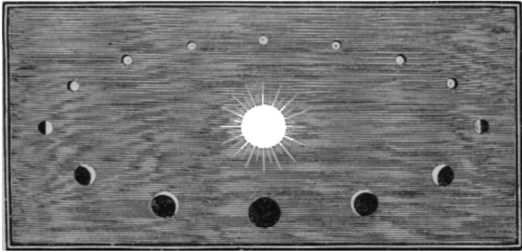
Fig. 108. – Ordine delle fasi di Venere.
