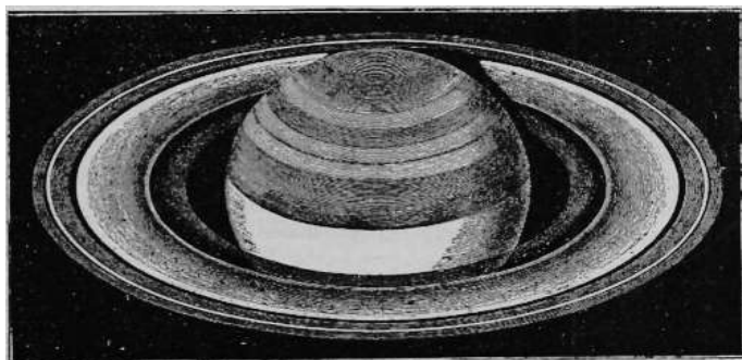
Fig. 284. – Saturno e i suoi anelli.
