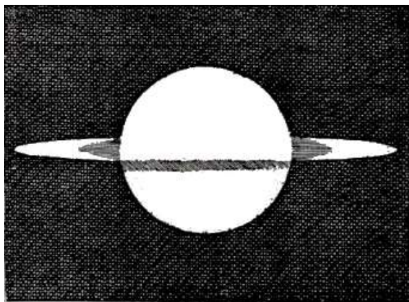
Fig. 286. – Primi disegni dell'anello di Saturno: HUYGENS, 1656.
