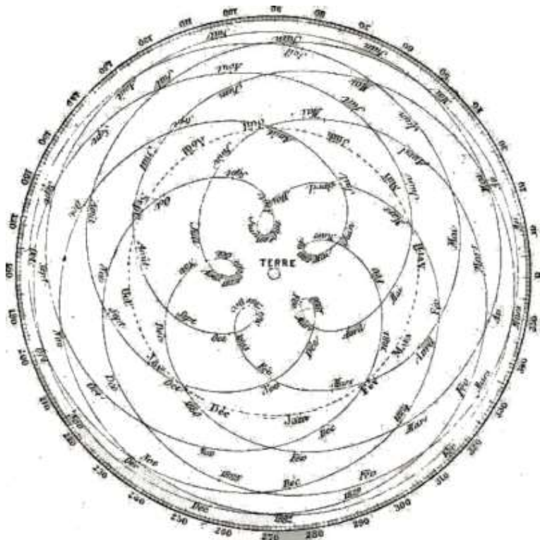
Fig. 40. – Moto di Marte in rapporto alla Terra.
