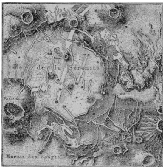
Fig. 222. – Topografia lunare: il mare della Serenità e il tumulo Linneo.
