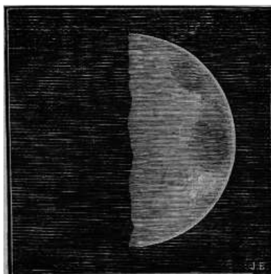
Fig. 112. – La Luna vista ad occhio nudo. Venere osservata col cannocchiale (4 febbraio 1883).
