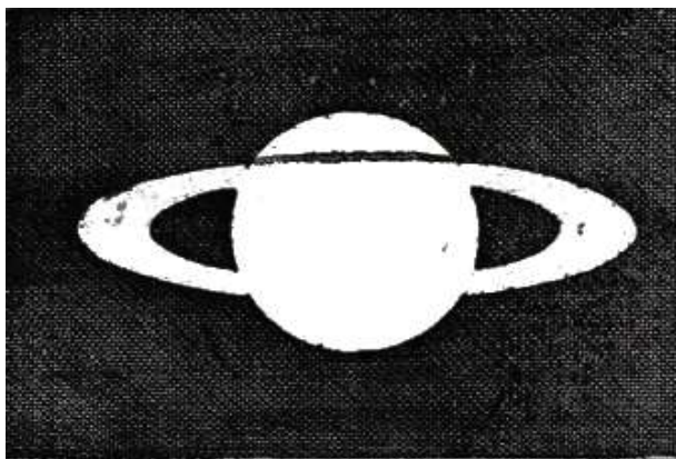
Fig. 288. – Primi disegni dell’anello di Saturno: HUYGENS, 1659.
