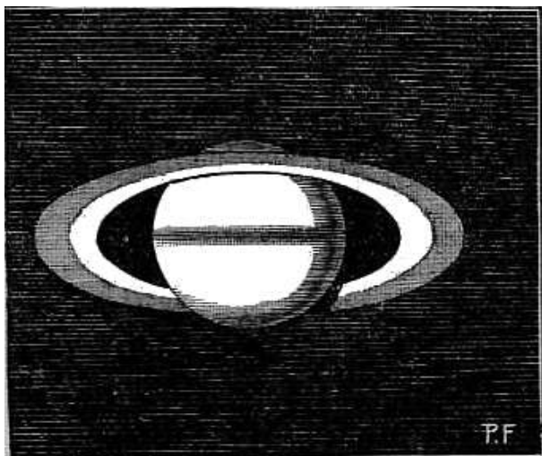
Fig. 290. – Primo disegno di una linea di separazione tra gli anelli: CASSINI, 1675.
