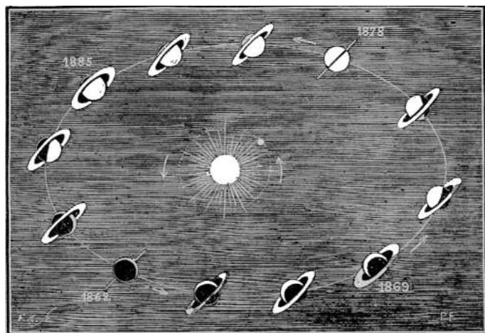
Fig. 293. – Prospettiva variabile degli anelli di Saturno visti dalla Terra.
