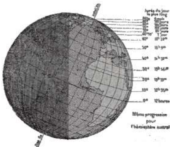
Fig. 181. – La Terra nel solstizio di giugno: durata del giorno secondo le latitudini.
