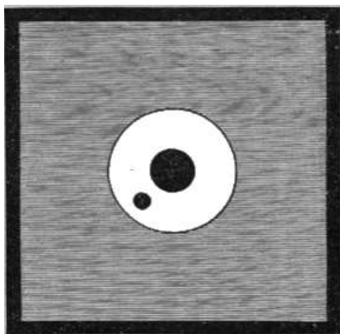
Fig. 79. – Passaggio della Terra e della Luna davanti al Sole, avvenuto per gli abitanti di Marte il 12 novembre 1879.
