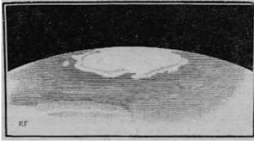
Fig. 68. – Le nevi del Polo Sud di Marte (1° settembre 1877). Fig. 69. – Le nevi del Polo Sud di Marte (10 settembre 1877).
