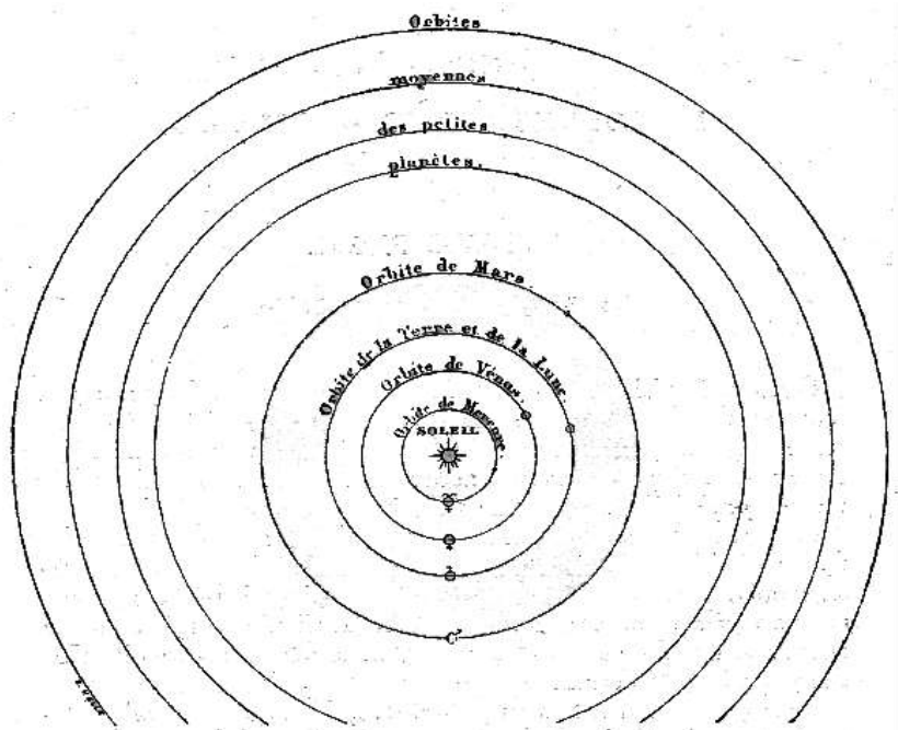
Fig. 179. – Orbita della Terra e dei pianeti vicini (scala 1 mm = 2 milioni di leghe)
