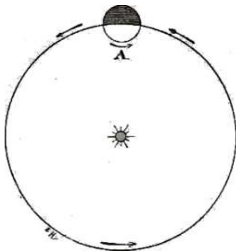
Fig. 246. – Paragone della velocità orbitale di Giove con la sua velocità di rotazione.
