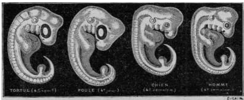
Fig. 89. – Le origini dell’uomo: embrioni comparati.
