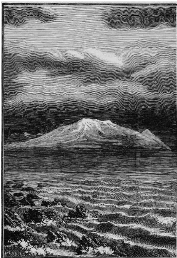
Fig. 63. – L'isola nevosa vista dall'Oceano Kepler: meteorologia marziana.
