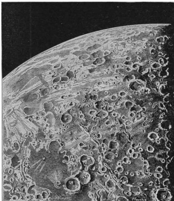
Fig. 204. – Regione montagnosa al sud del mare della Fecondità.
