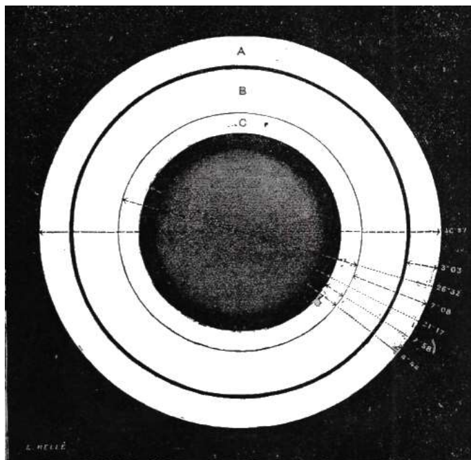
Fig. 296. – Il sistema di Saturno (misure di Meyer, 1880).
