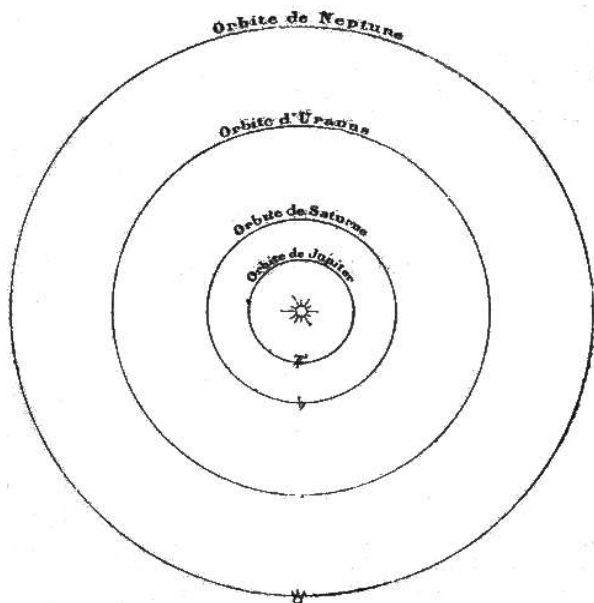
Fig. 320. – I mondi principali del sistema solare (scala: 1 mm. = 20 milioni di leghe).
