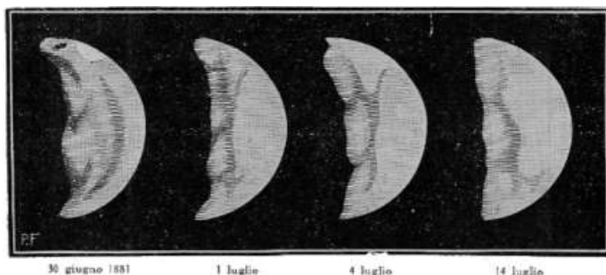
Fig. 131. – Aspetti telescopici del pianeta Venere: disegni di Niesten.
