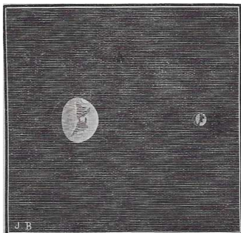
Fig. 147. – Aspetto della Terra e della Luna viste da Venere.
