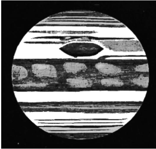
Fig. 251. – Aspetto di Giove il 7 dicembre 1881.
