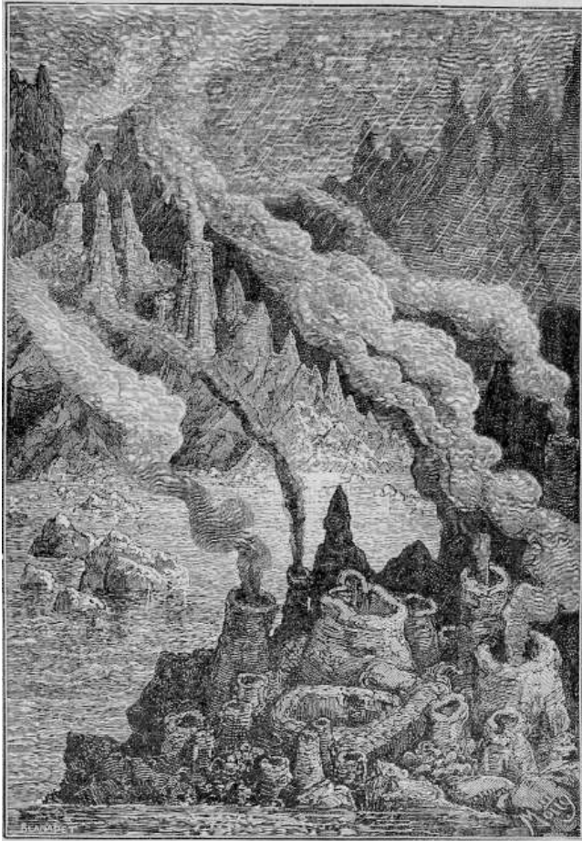
Fig. 227. – I geysers di fango dell'Islanda danno forse un'idea di ciò che accadeva allora sulla Luna.
