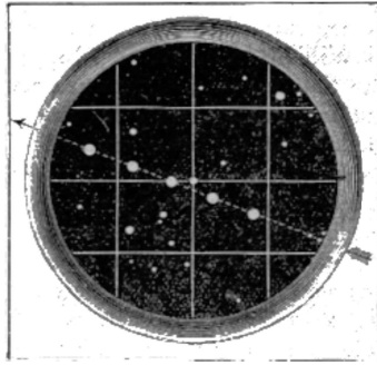
Fig. 235 – Come si trovano i piccoli pianeti.
