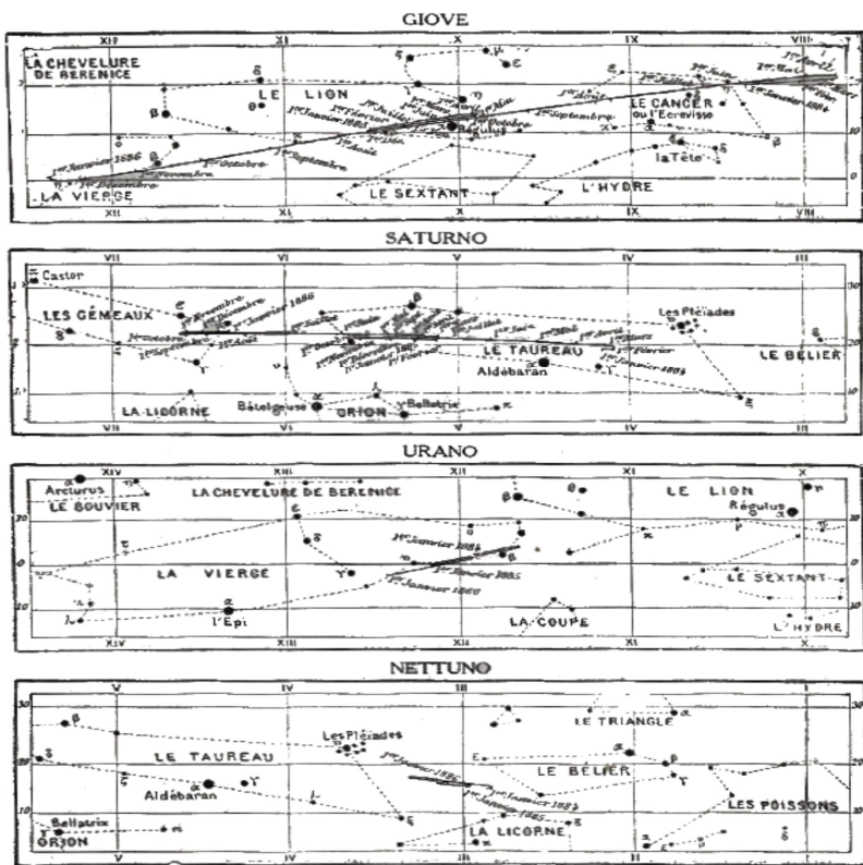
Fig. 269. – Moto e posizioni dei pianeti Giove, Saturno, Urano e Nettuno durante due anni (1884 e 1885).
