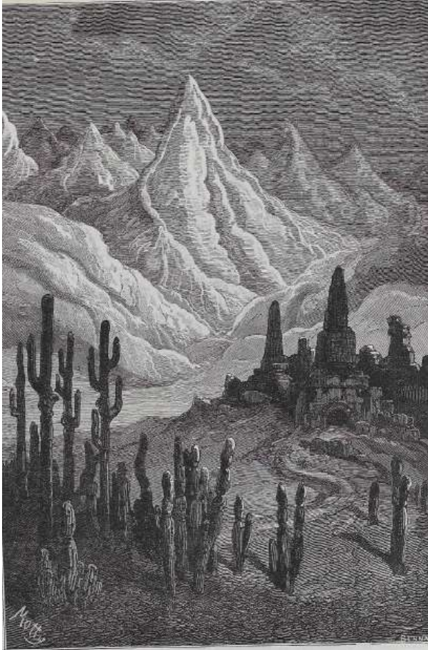
Fig. 145. – ... Forse non saremmo troppo smarriti arrivando davanti a un paesaggio di Venere.
