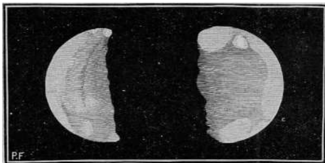
Fig. 130. – Aspetti telescopici del pianeta Venere, da Gruithuisen.
