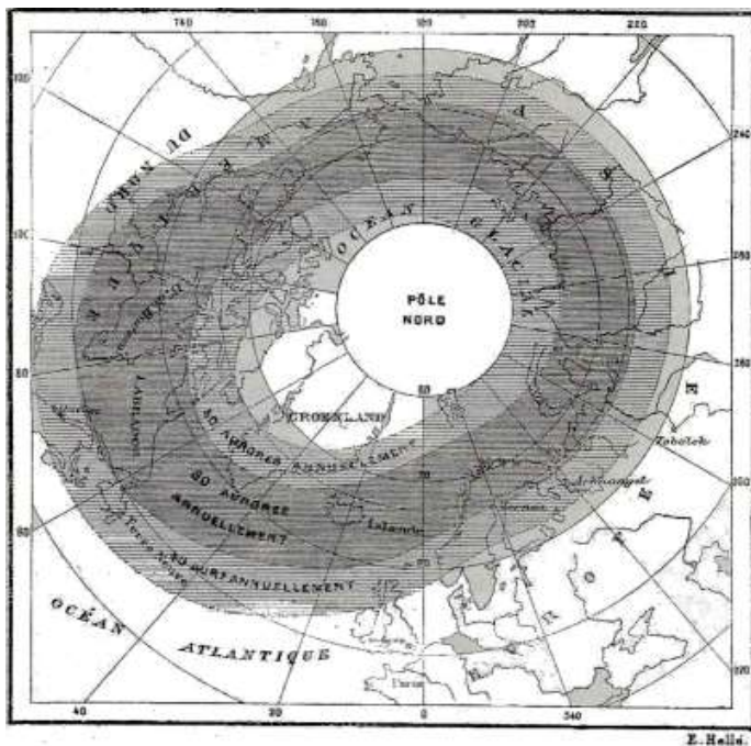
Fig. 191. – Distribuzione circumpolare delle aurore boreali.
