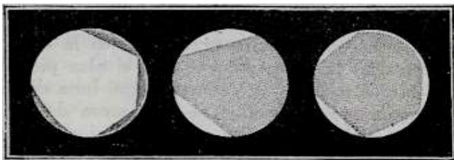
Fig. 267. – Aspetti osservati sul quarto satellite di Giove.
