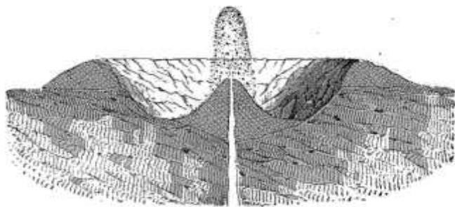
Fig. 214. – Sezione geologica d'un vulcano lunare nel suo ultimo periodo d'attività.
