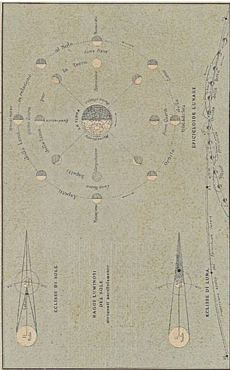
LA LUNA E LE SUE FASI.
