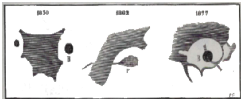
Fig. 25. – Variazioni osservate sul pianeta Marte: il mare Terby nel 1830, 1862 e 1877.
