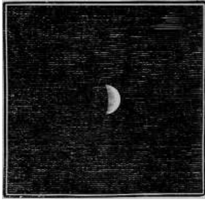
Fig. 92. – Aspetto della Terra vista da Marte (giugno 1884).
