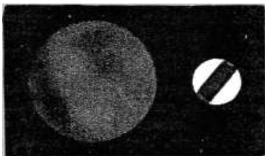
Fig. 166. – Grandezza comparata di Mercurio e della Terra.
