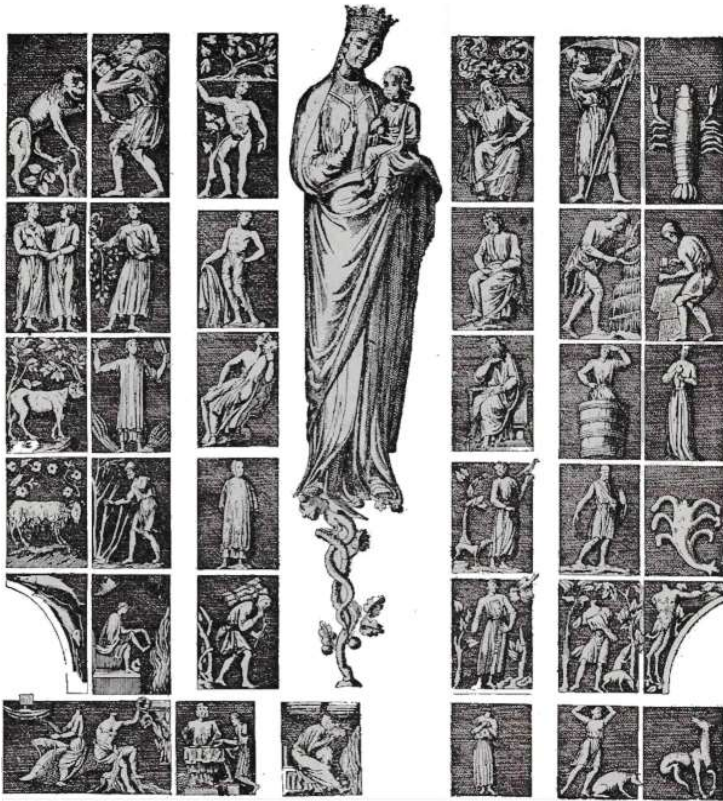
Fig. 278. – Zodiaco scolpito nella facciata di Nostra Signora di Parigi.
