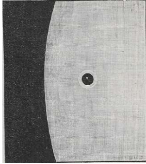
Fig, 168. – Aureola luminosa osservata intorno a Mercurio
