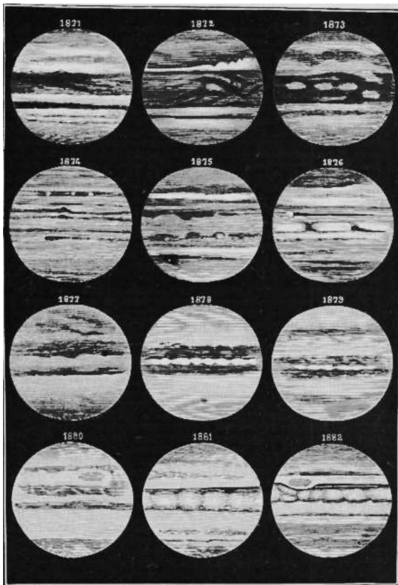
Fig. 254. – Aspetto telescopico di Giove durante 12 anni.
