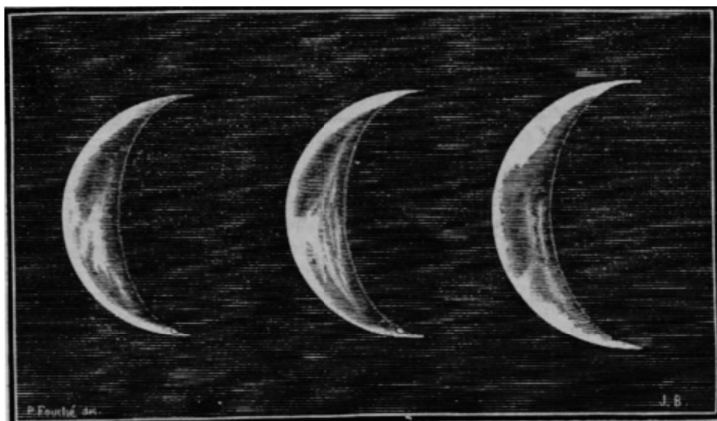
Fig. 128. – Aspetti geografici del pianeta Venere. (Disegni di Denning, 1881.)
