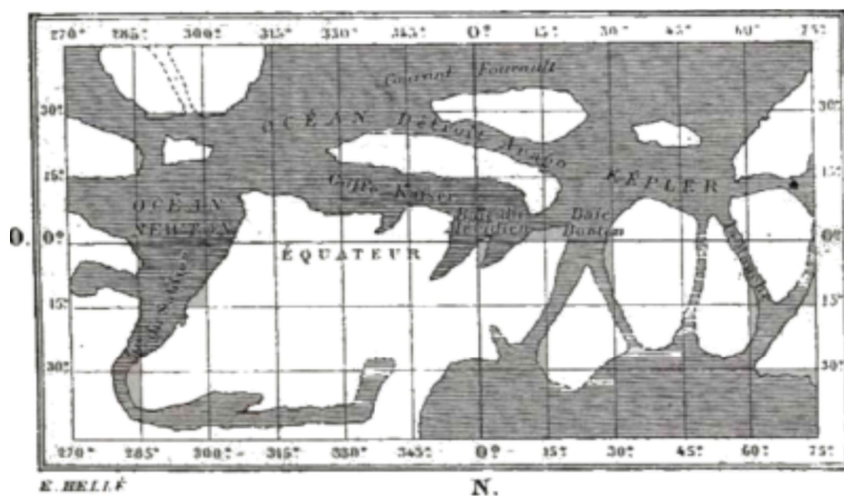
Fig. 19. – Geografia di Marte: la Baia del Meridiano.
