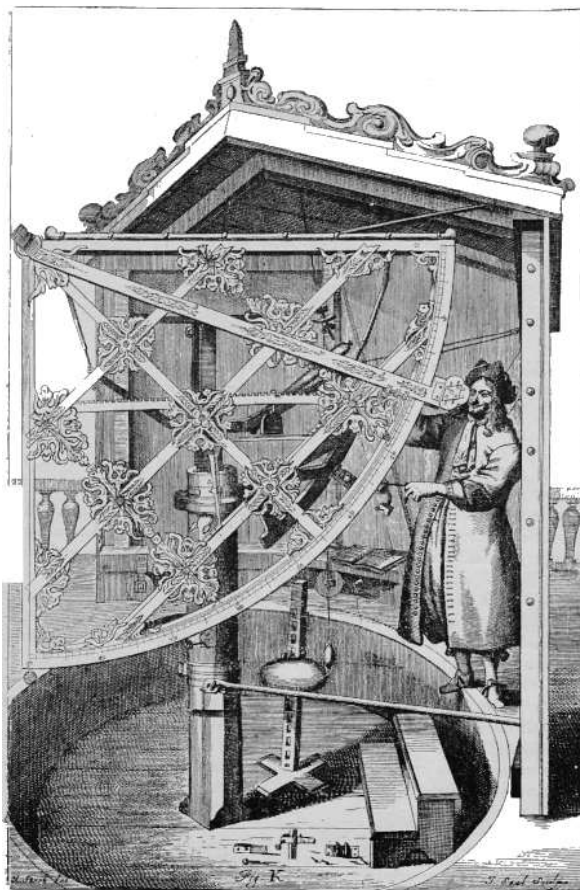
Fig. 56. – Strumenti astronomici del tempo d'Hevelius.
