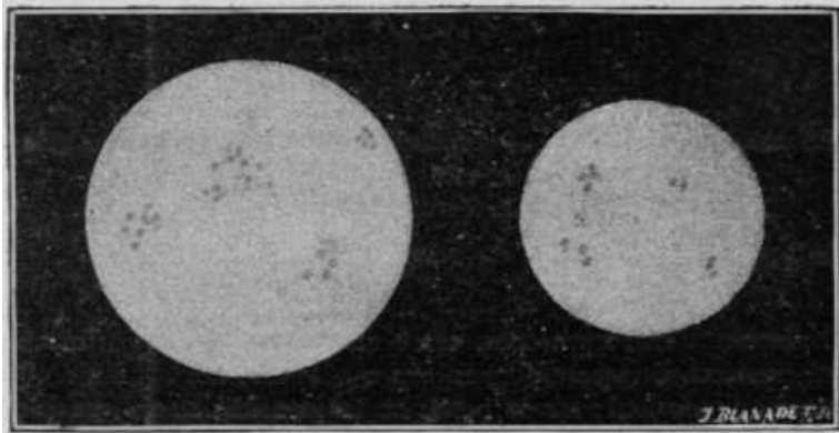
Fig. 142. – Grandezza comparata del Sole visto da Venere e visto dalla Terra (scala 1^{\text{mm}} = 1' )
