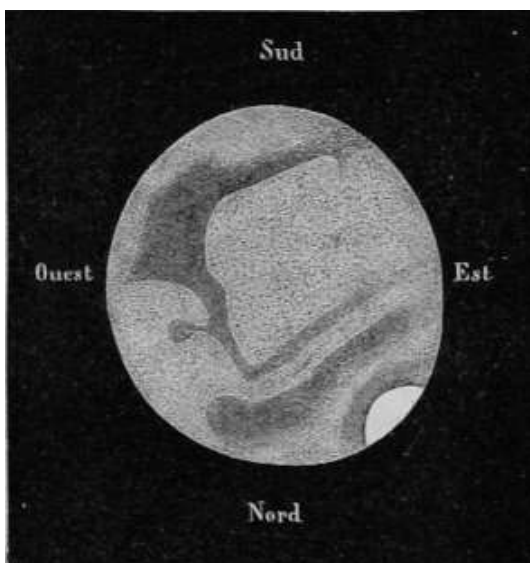
Fig. 51. – Le stagioni di Marte: aspetto del pianeta il 29 giugno 1873.
