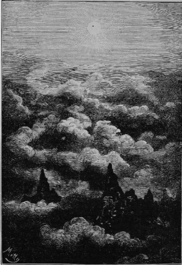
Fig. 259. – Vista da Giove, la Terra non è che un minuscolo punto nero dinanzi al Sole.
