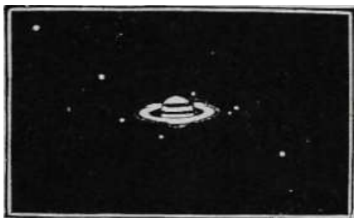
Fig. 299. – Il corteo di Saturno (i primi otto satelliti).
