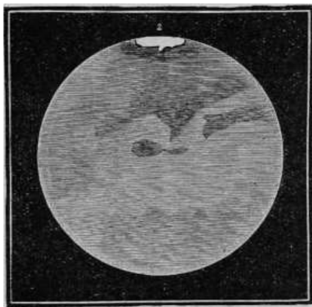
Fig. 65. – Aspetto di Marte il 29 settembre 1877, alle nove di sera.
