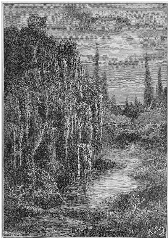
Fig. 196. – La sua luce scende come un sogno sul sonno della natura.
