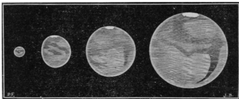
Fig. 43. – Le fasi di Marte.
