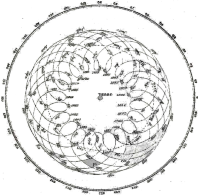
Fig. 156. – Movimento di Mercurio in rapporto alla Terra.
