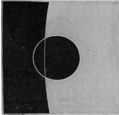
Fig. 137. – L'aureola atmosferica di Venere (Orgères, 6 dicembre 1882).
